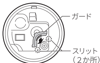
本体(上から見た図)
